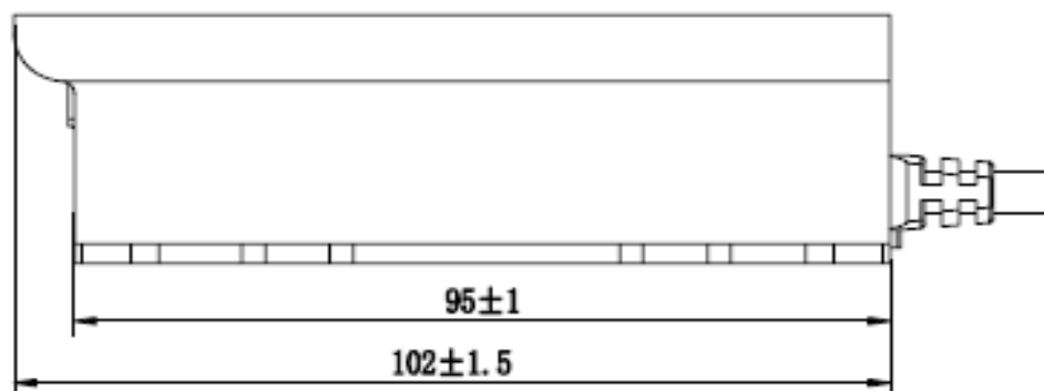
Вид слева
