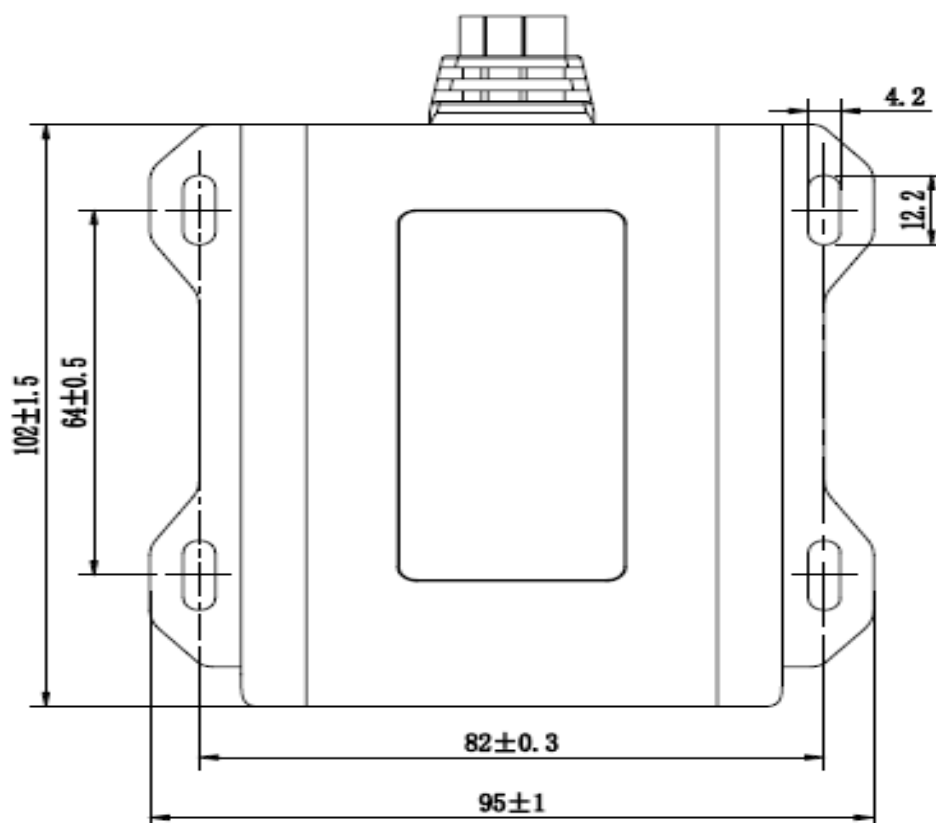
Вид сверху
