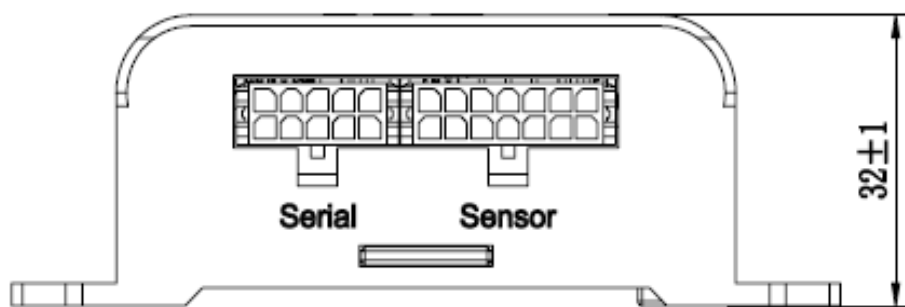
Вид спереди
